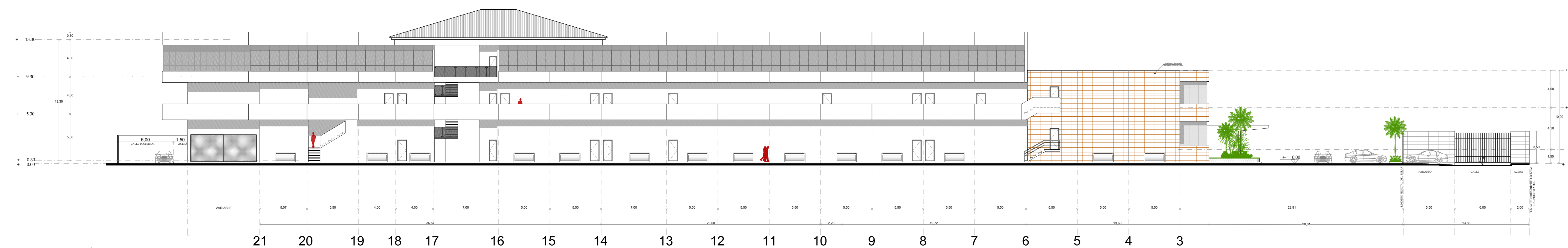
PROYECTO ARQUITECTÓNICO ALZADO LATERAL FACHADA ESTE ESCALA 1-200
