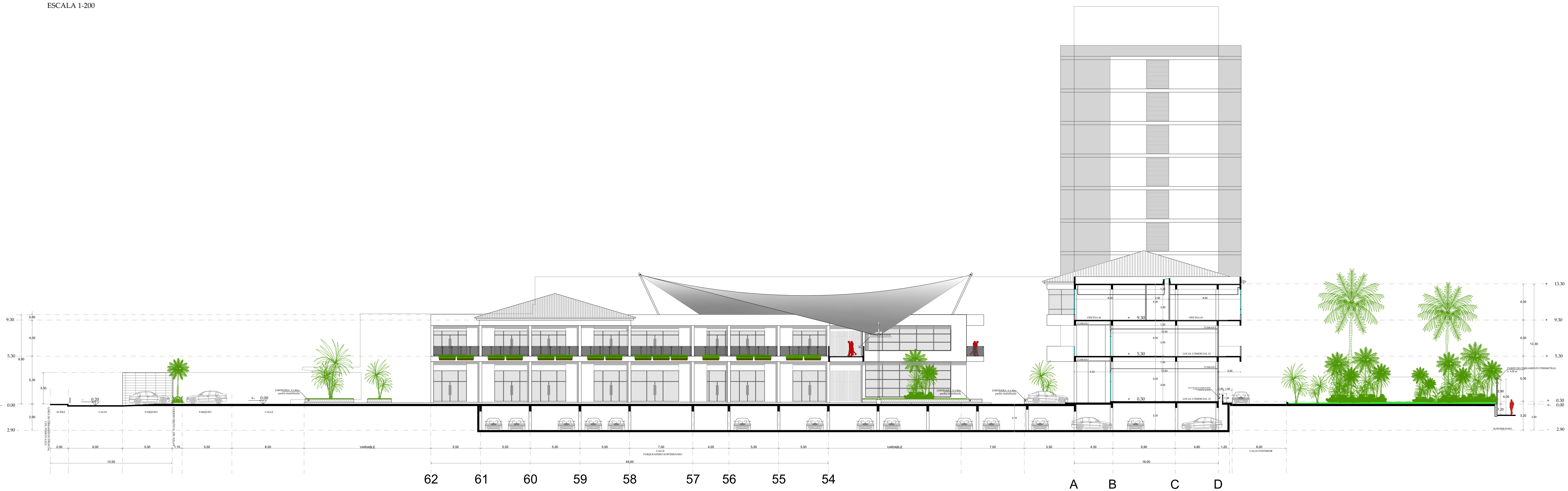
PROYECTO ARQUITECTÓNICO CORTE F-F' ESCALA 1-200
