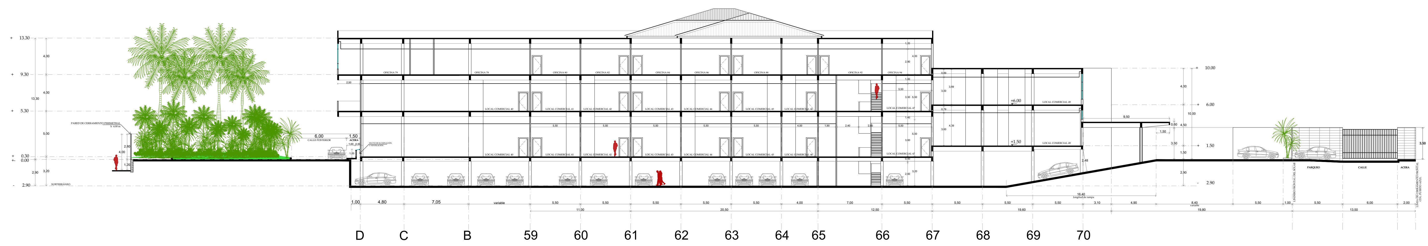
PROYECTO ARQUITECTÓNICO CORTE D-D' ESCALA 1-200
