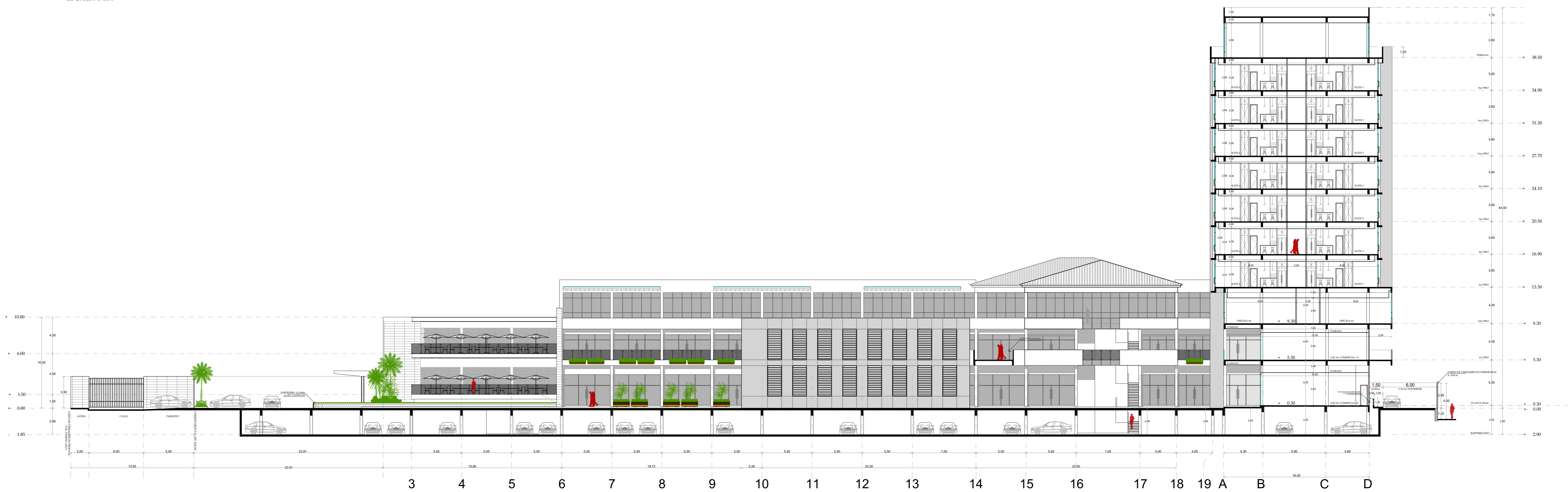
PROYECTO ARQUITECTÓNICO CORTE B-B' ESCALA 1-200
