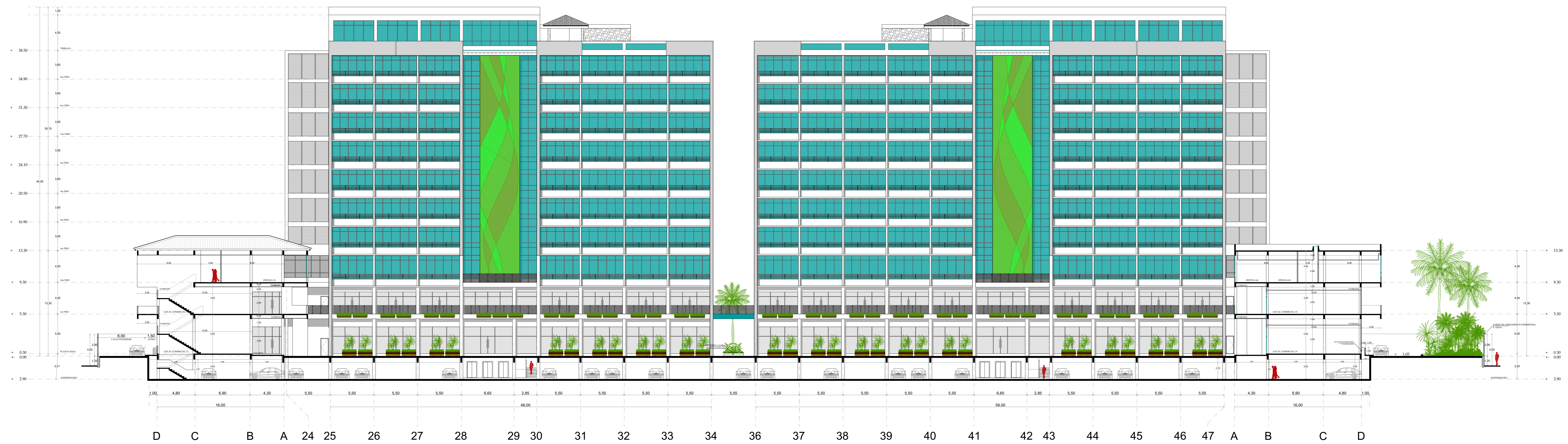
PROYECTO ARQUITECTÓNICO CORTE A-A' ESCALA 1-200
